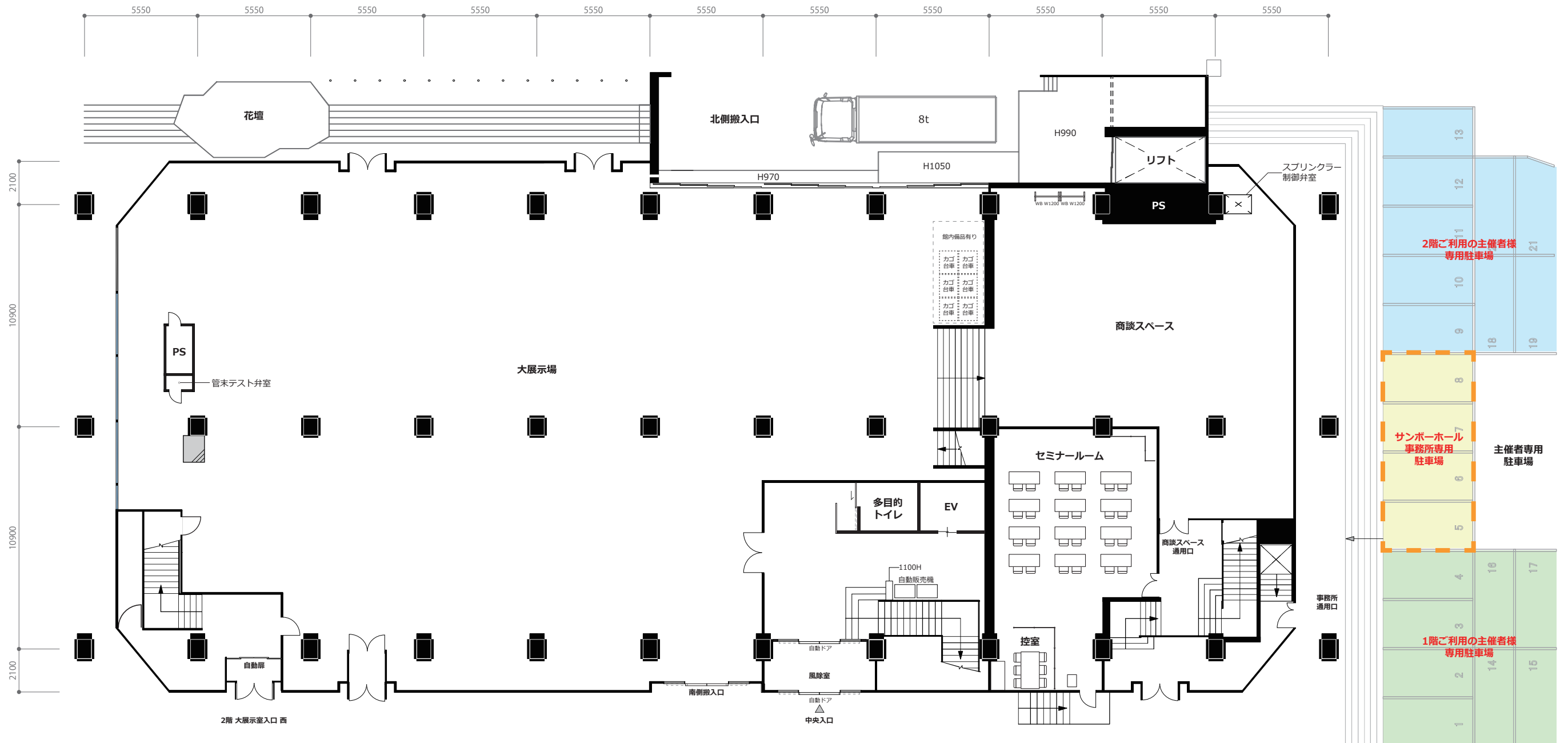
神戸サンポートホール 1階 平面・立面図
